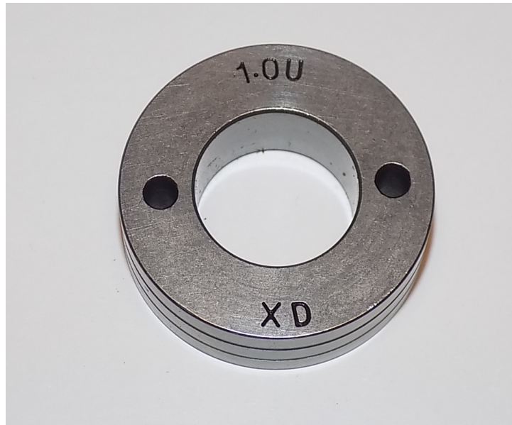
РОЛИК ПОДАЮЩИЙ ПОД АЛЮМИНИЙ (37-19-12) 0,8/1.0
